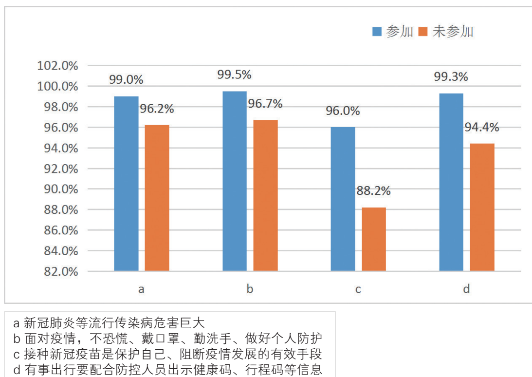
图5 “青少年科技素养提升计划”课程不同参与情况下对有关疫情防控说法的赞同比例（单位：%）
