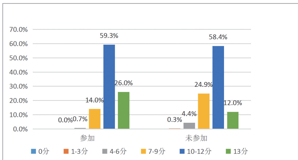
图2 “青少年科技素养提升计划”课程不同参与情况下的“科学原理”测试得分（单位：%）
