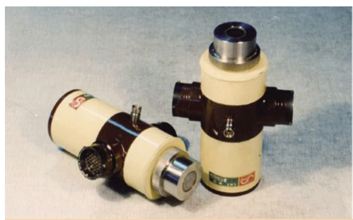
60像元长波红外探测器。
