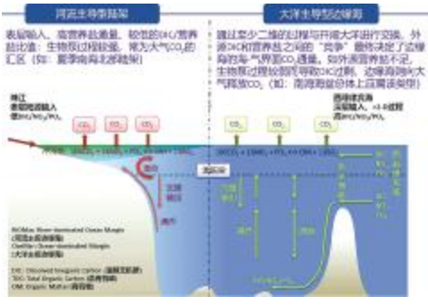
河流主导型陆架和大洋主导型边缘海的差别
