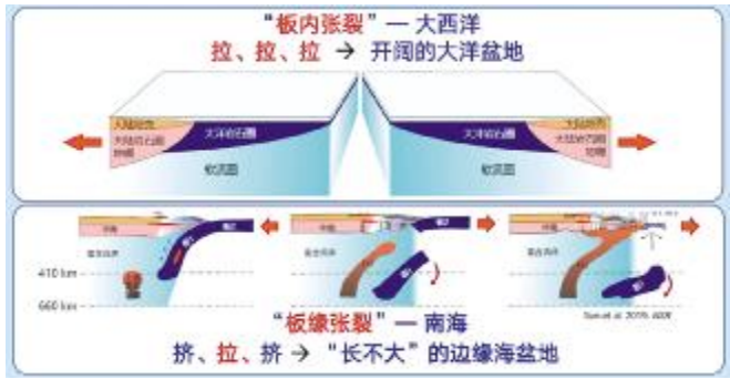
南海“板缘张裂”模式与大洋“板内张裂”的异同
